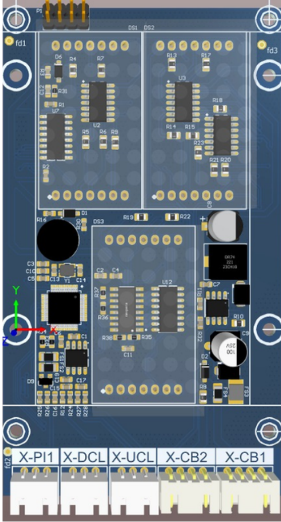
Görsel 1: BC-D3X Ön Yüzden 3D Görüntüsü
