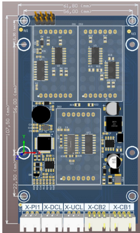
Görsel 3: BC-D3X Montaj Ölçüleri
