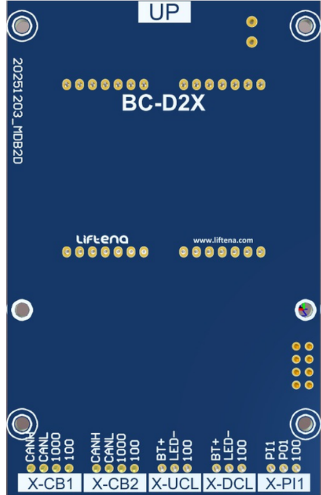
Görsel 2: BC-D2X Arka Yüzden 3D Görüntüsü
