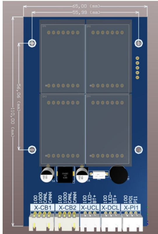
Görsel 3: BC-D2X Montaj Ölçüleri
